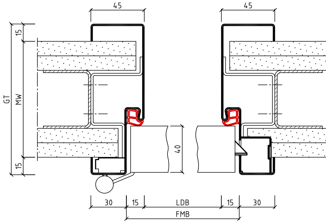
Horizontalschnitt
