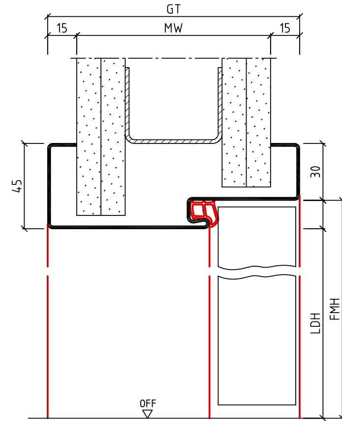
Vertikalschnitt
