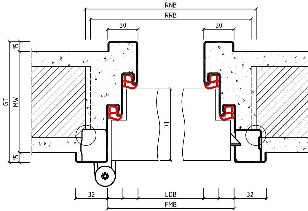
Horizontalschnitt
