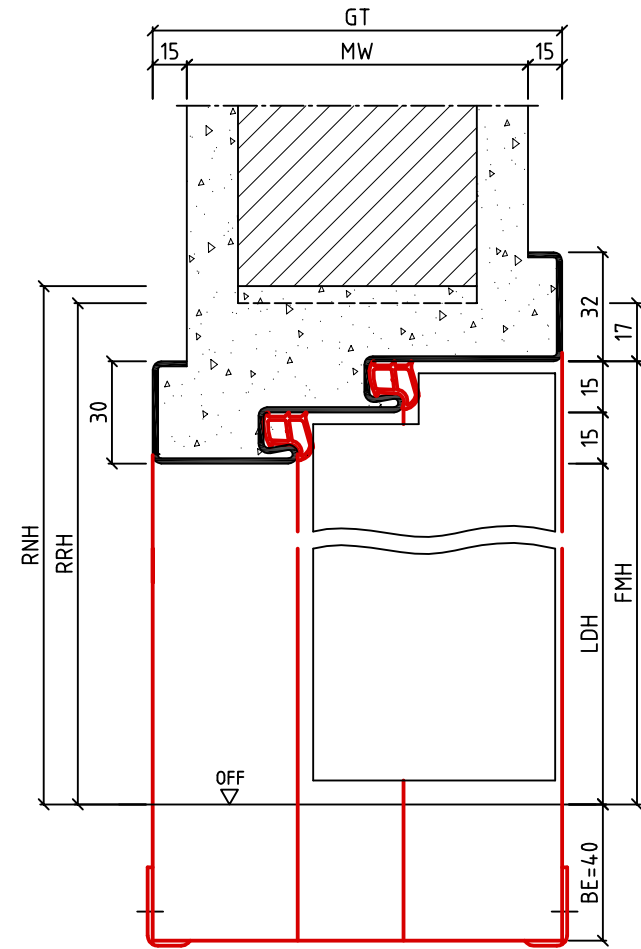
Vertikalschnitt
