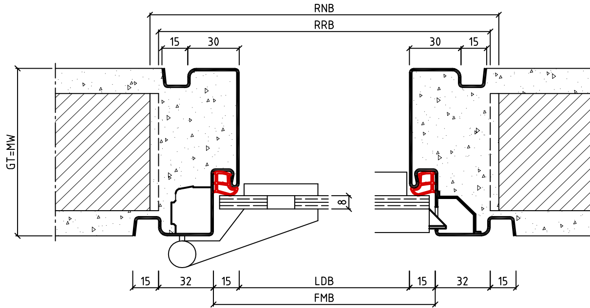
Horizontalschnitt
