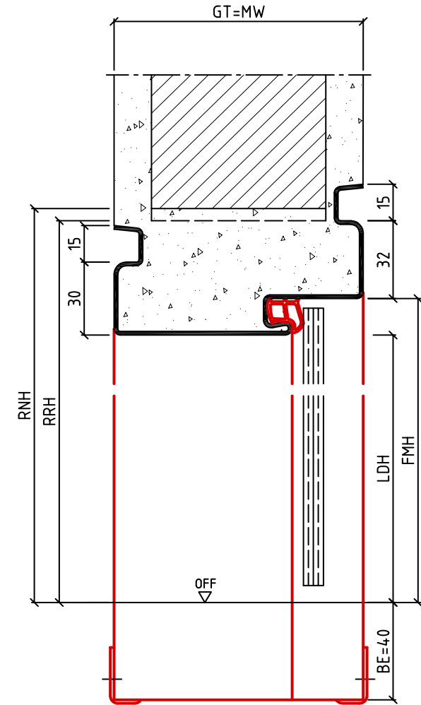
Vertikalschnitt
