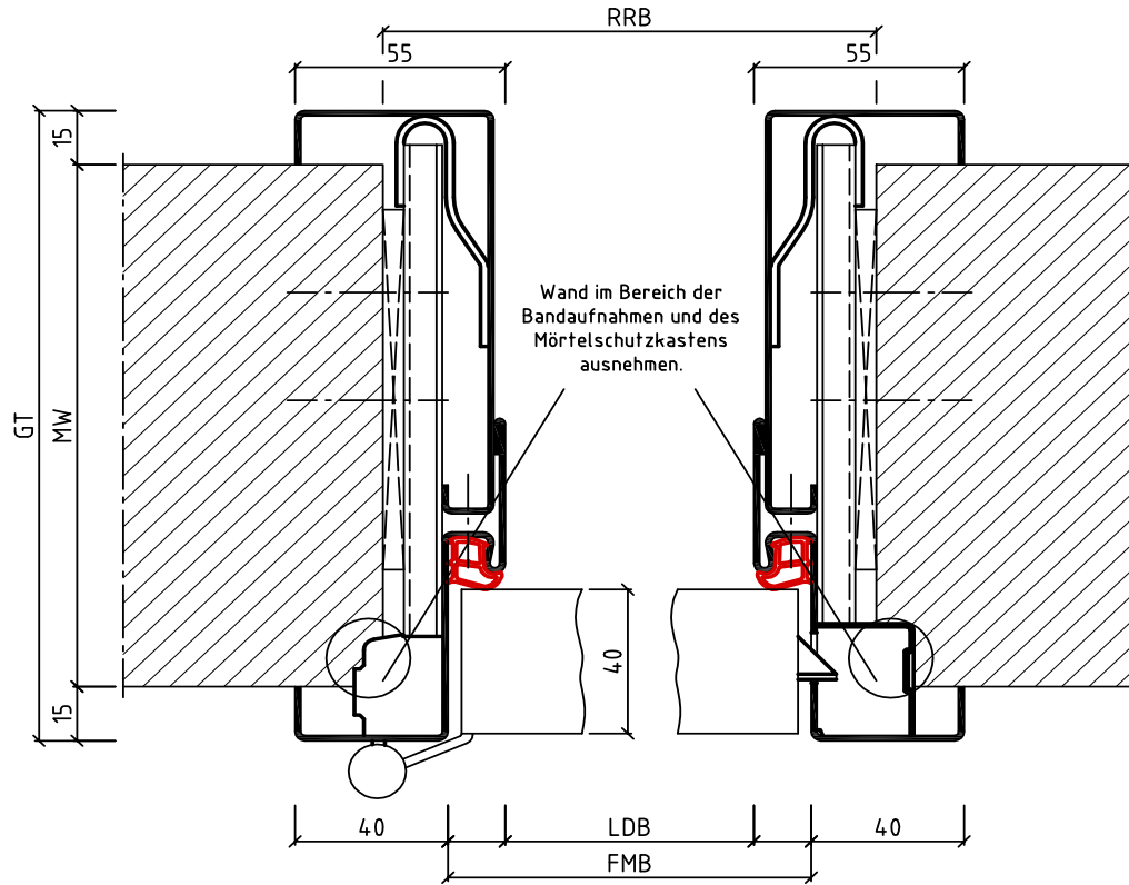
Horizontalschnitt
