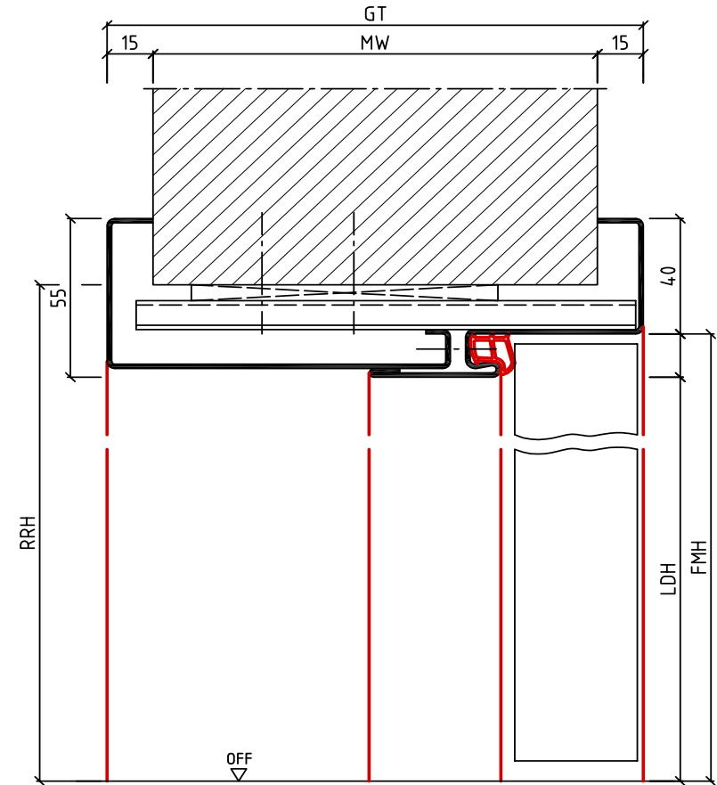
Vertikalschnitt
