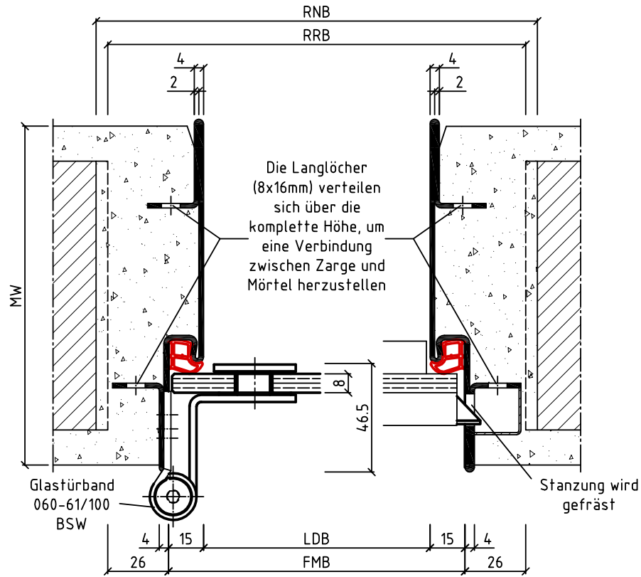
Horizontalschnitt
