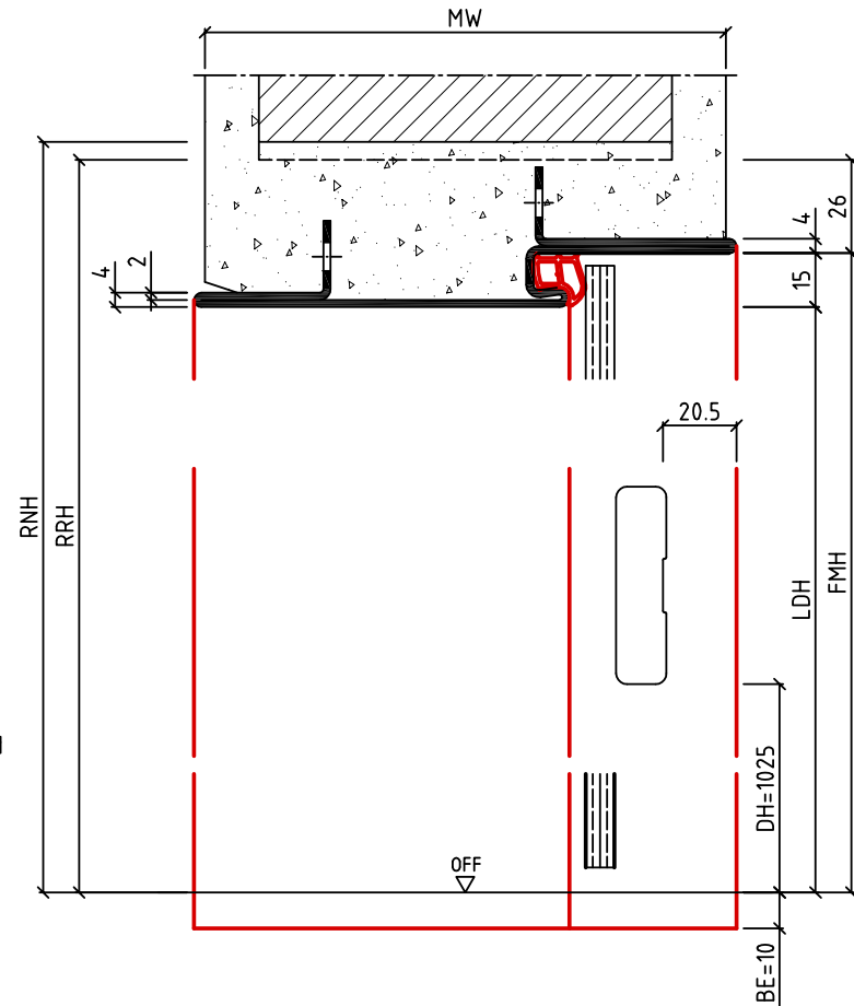
Vertikalschnitt
