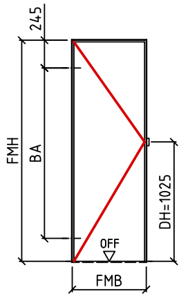
Ansicht: DIN links spiegelbildlich: DIN rechts
