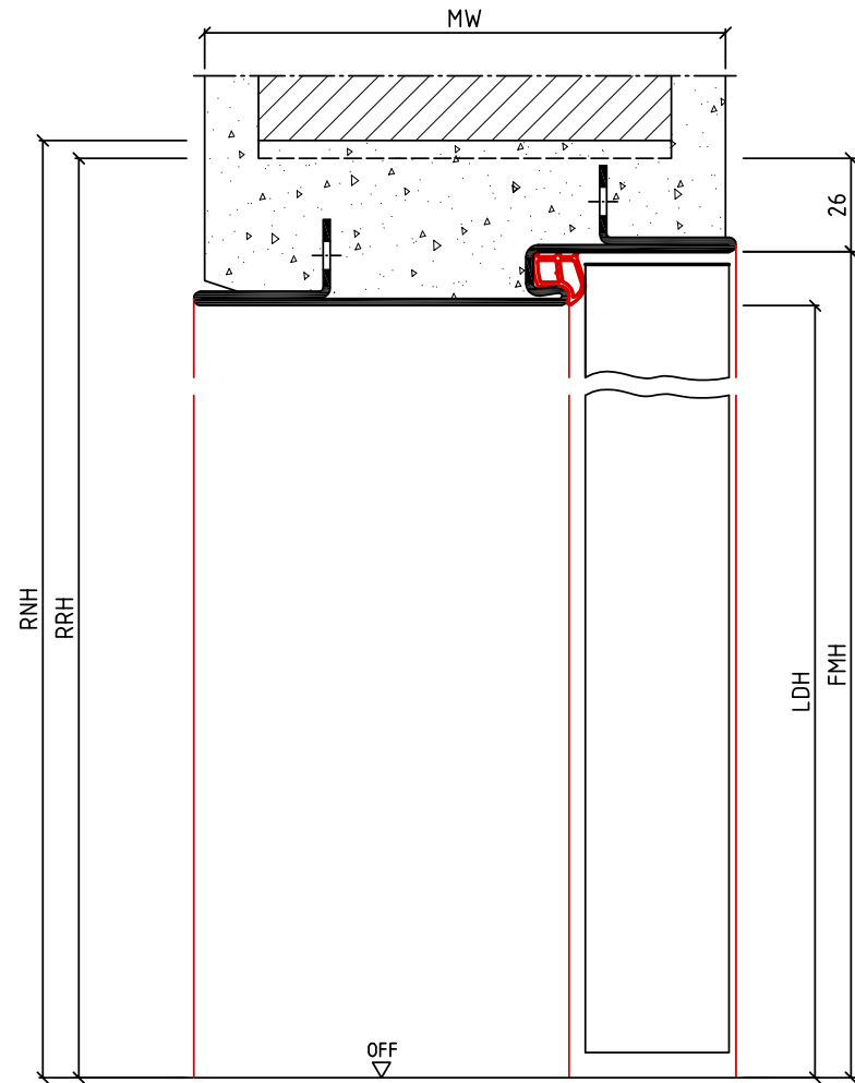
Vertikalschnitt
