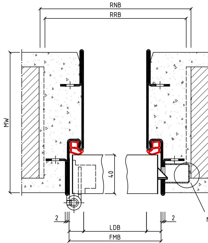
Horizontalschnitt
