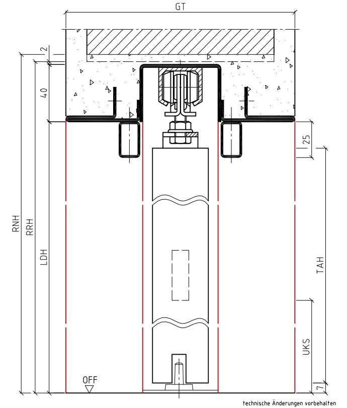
Vertikalschnitt
