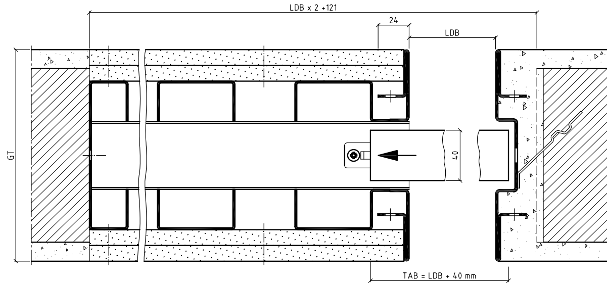
Horizontalschnitt
