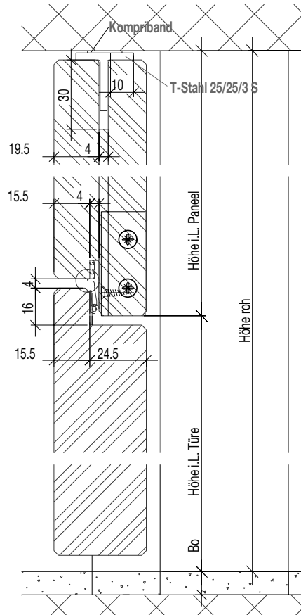
Schnitt A-A
