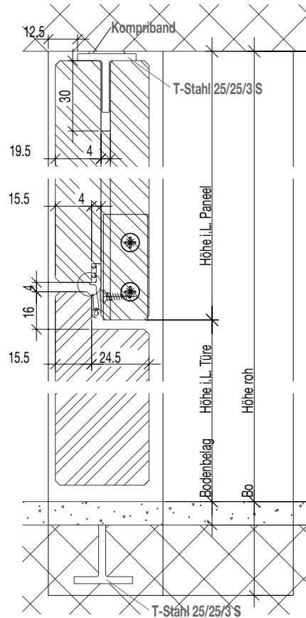
Schnitt A-A
