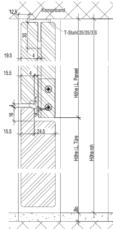
Schnitt A-A
