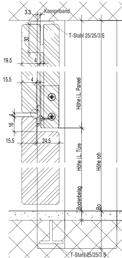
Schnitt A-A
